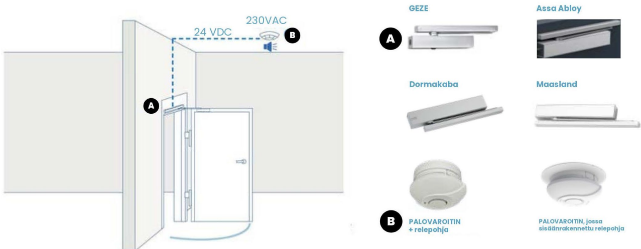
Kuva 2. FITO / NORDIC -palonsulkujärjestelmä valvoo tilaa ja sulkee oven automaattisesti hälytyksen yhteydessä
